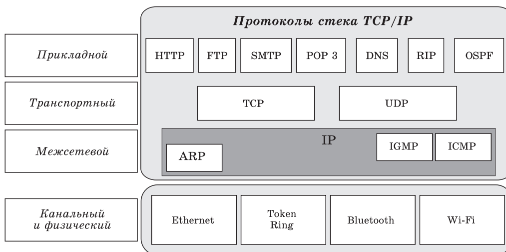
Рис. 7.1. Основные протоколы стека TCP/IP
